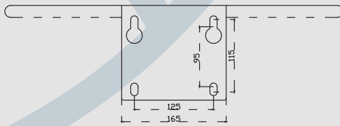
ÇEMBER DELİK MERKEZLERİ
